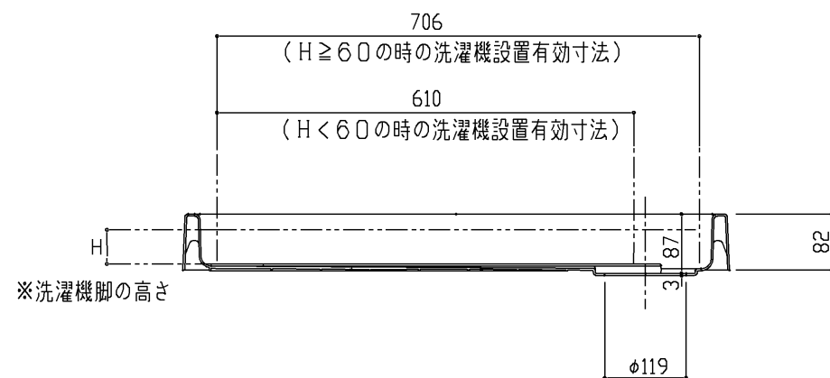
断面A-A
